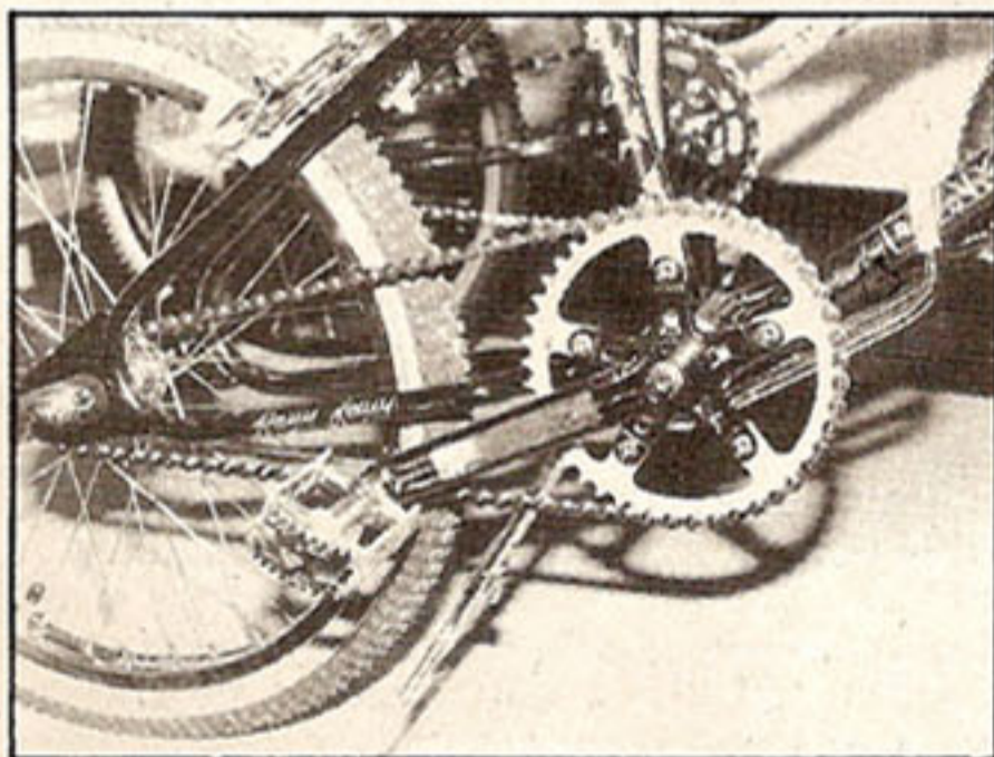
Sur le Diamond Back « Turbo » qui se trouve au sommet de la gamme, on découvre ce pédalier dural original. Le gros boîtier est équipé de roulement protégés de la poussière ; les manivelles forgées sont de pures merveilles de finition. Naturellement, le plateau dural est interchangeable.
