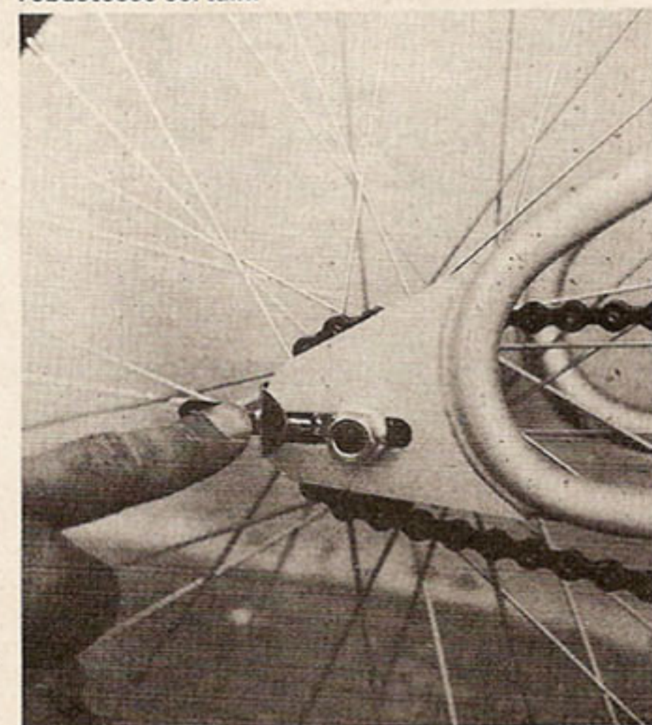
La partie postérieure du cadre est pourvue de tendeurs de chaîne. Ils gagneraient à posséder des repères pour faciliter l'alignement de la roue.
