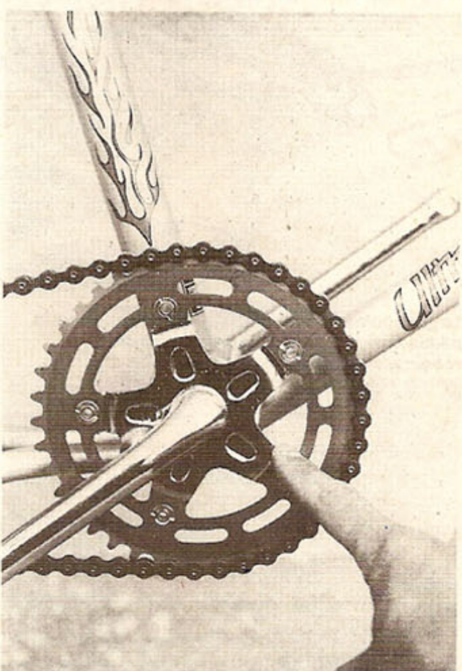
Le moyeu du pédalier est en acier. La couronne est toutefois en dural.
